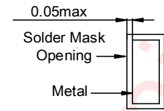
Non Solder Mask Define
