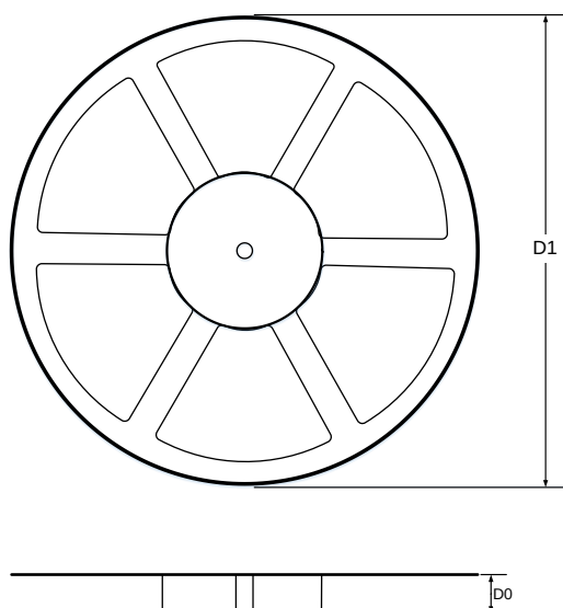
REEL DIMENSIONS
