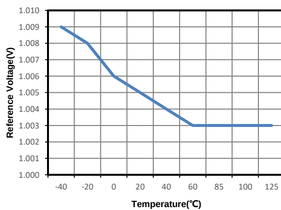
VREF vs TEMP
